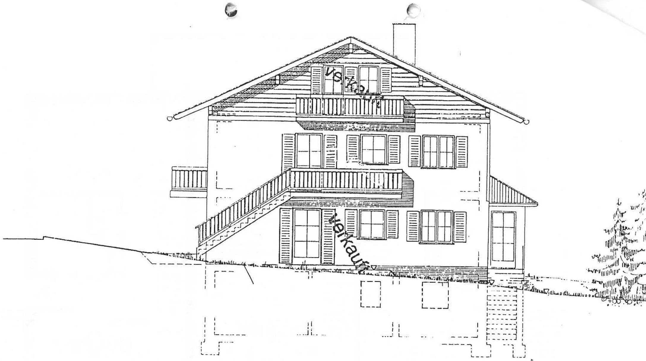
OST - ANSICHT
